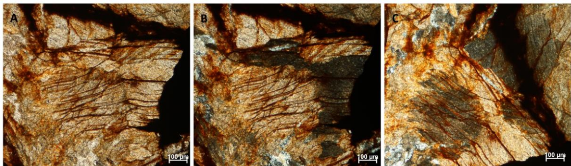
Slika 27: Fotomikrografija uzorka B2 s kremenom, sideritom i opakim mineralima u prolaznoj svjetlosti: A) bez uključenog analizatora, B) s uključenim analizatorom, C) s uključenim analizatorom u položaju maksimalnog potamnjenja.
