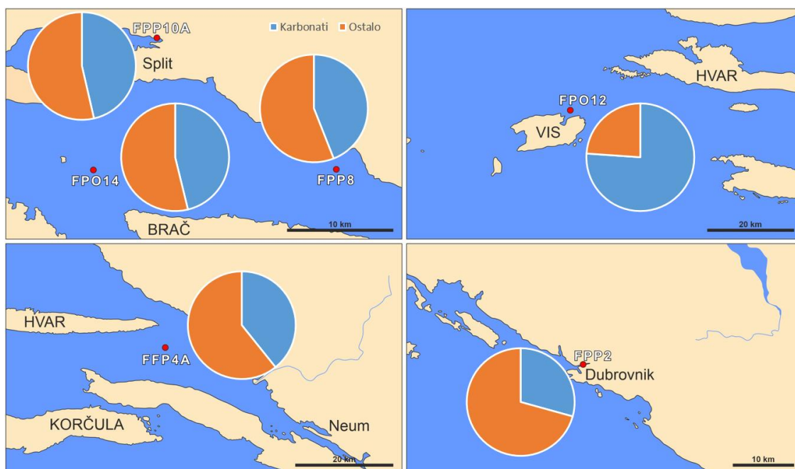
Slika 14 - Odnos udjela karbonata pojedinih uzoraka na geografskom prikazu
