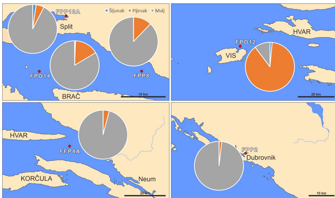
Slika 13 - Odnos granulometrijskih frakcija pojedinih uzoraka na geografskom prikazu
