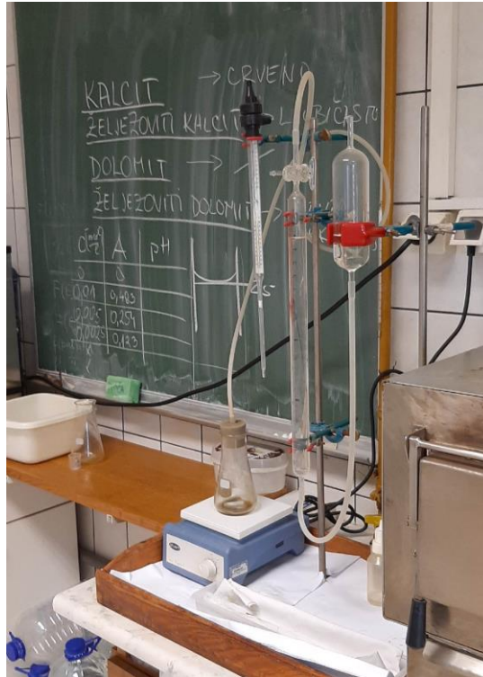
Slika 5 - Aparatura za calcimetriju
