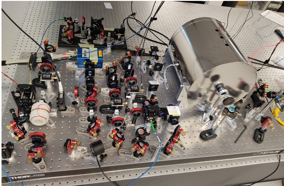
Slika 3.1: Eksperimentalni postav.
