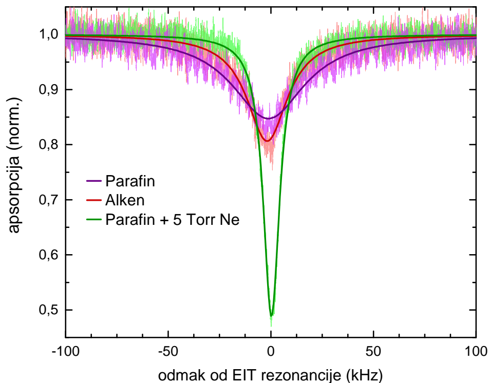
Slika 4.1: Apsorpcijski spektar EIT-a triju mjerenih ćelija za istu snagu pumpne zrake na sobnoj temperaturi. Jasno je vidljivo da je najuža EIT rezonancija ona mjerena na ćeliji koja sadrži neon i parafinski premaz. Ćelije iznutra premazane parafinom i alkenom su sličnije, ali je očito da ćelija premazana alkenom ima užu rezonanciju EIT-a.
