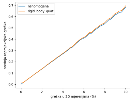
Slika 5.6: Rezultati testa otpornosti metode gradijentnog spusta s parametrizacijom kvaternionima na pogrešku u mjerenju s kardinalitetima stanja 5, 10 i 20. Metrika m_2 prikazana je u lijevom stupcu, a srednja reprodukcijaska greška u desnom.
