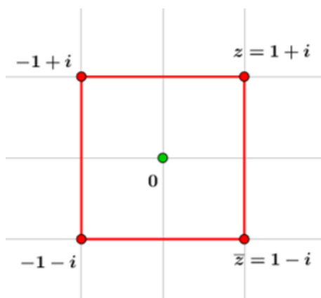
Slika 4.4: Razgranati primagon
