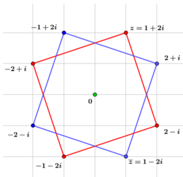
Slika 4.5: Podijeljeni primagon
