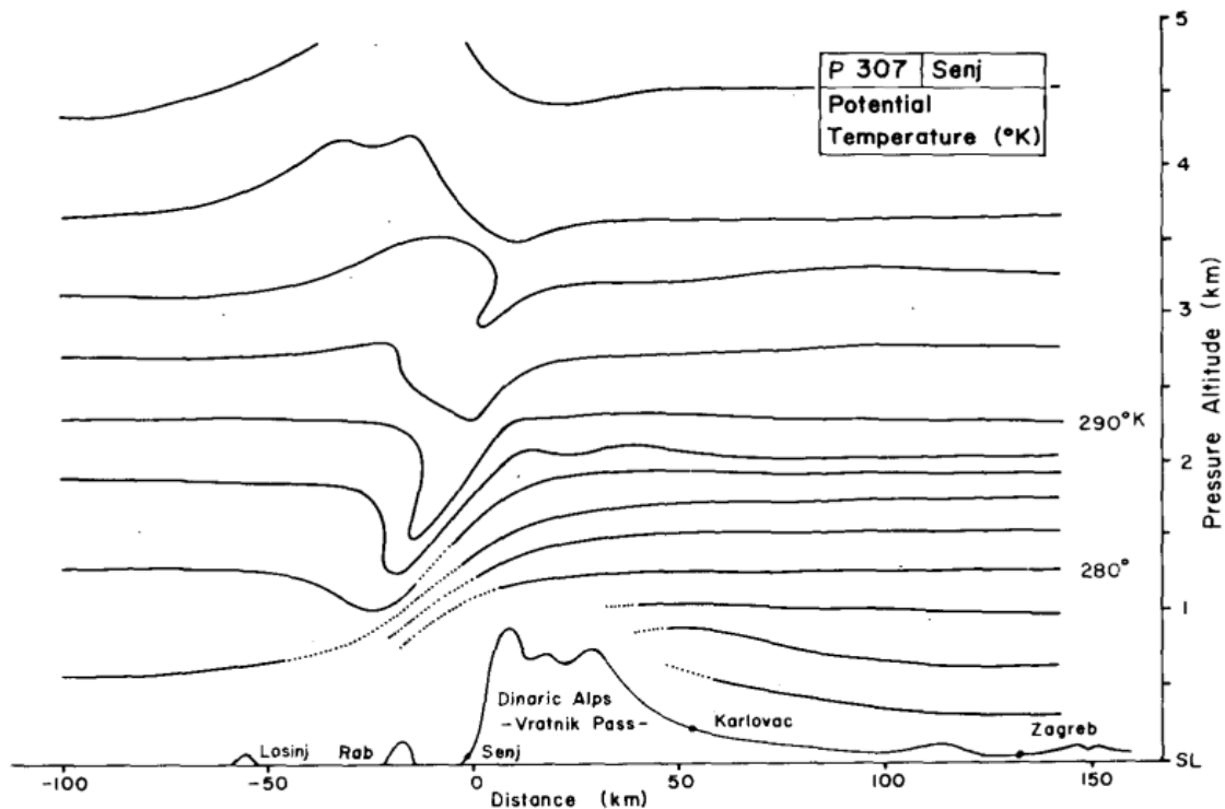
Slika 1.3. Vertikalni presjek za jedan termin puhanja bure kod Senja - izentropole. (Preuzeto iz Smith, 1987; slika 6b)
