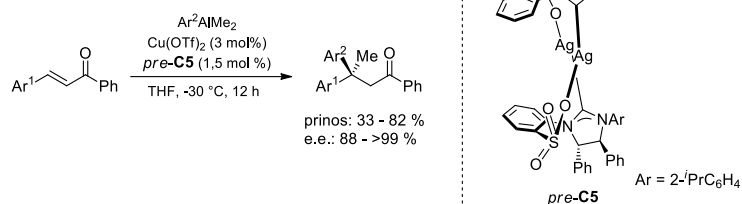
Slika 15. Shematski prikaz priprave \beta,\beta -diaril ketona konjugiranom adicijom arilaluminijevih spojeva na \beta -aril- \beta,\beta -disupstituirane acikličke enone u prisutnosti bakrovog katalizatora
