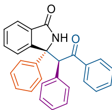
( R )-3-(( S )-2-okso-1,2-difeniletel)-3-fenilizoindolin-1-on (( 3R,S )- 41 )
