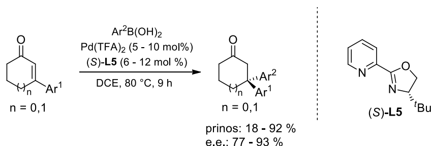
Slika 16. Shematski prikaz priprave \beta,\beta -diaril ketona adicijom arilborne kiseline na cikličke enone katalizirane kataliziranom paladijevim katalizatorom
