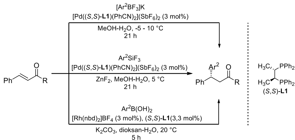
Slika 8. Stereoselektivna adicija kalijevo ariltrifluorborata, 51,52 ariltrifluorsilana 52 i arilboronične kiseline 53 na izabrane acikličke enone u prisutnosti kiralnih kompleksa prijelaznih metala
