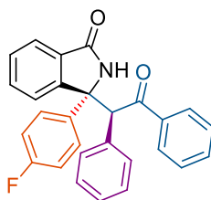
( R )-3-(4-fluorfenil)-3-(( S )-2-okso-1,2-difeniletil)izoindolin-1-on ((3 R,S )- 46 )
