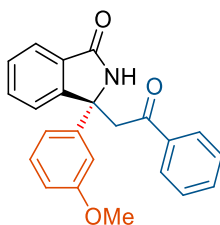
( R )-3-(3-metoksifenil)-3-(2-okso-2-feniletil)izoindolin-1-on (( R )- 23 )
