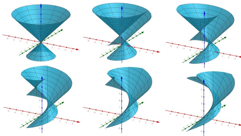
Slika 2.1: Plohe iz asocirane familije svjetlosnog stošca za t \in \{0, 0.25, 0.5, 0.75, 1, 1.25\}
