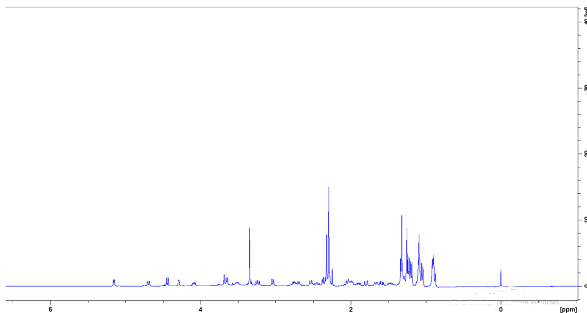
Slika 28. Spektar ^1\text{H} NMR spoja M4'' snimljen u kloroformu-d pri 298K.
