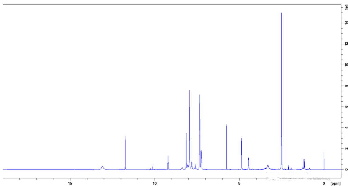
Slika 9. Spektar ^1\text{H} NMR tiosemikarbazona P6 snimljen u \text{DMSO-d}_6 pri 298K.
