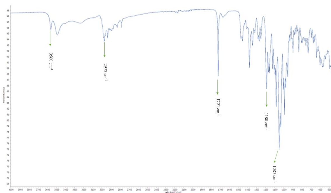
Slika 19. Snimljeni spektar IR azitromicina. Vrpce istežanja pri 3560 cm -1 [ν(O-H)], 2972 cm -1 [ν(CH 2 )], 1721 cm -1 [ν(C=O)], 1188 cm -1 [ν(R-O-R)], 1087cm -1 [ν(C-N)] potvrđuju strukturu azitromicina.
