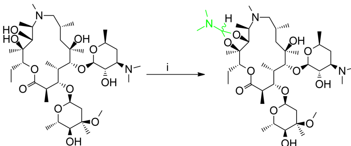
Schema 8. (i) N,N -Dimetilformamid-dimetilacetal (DMF-DMA), toluen, 60 °C, 24 h.
