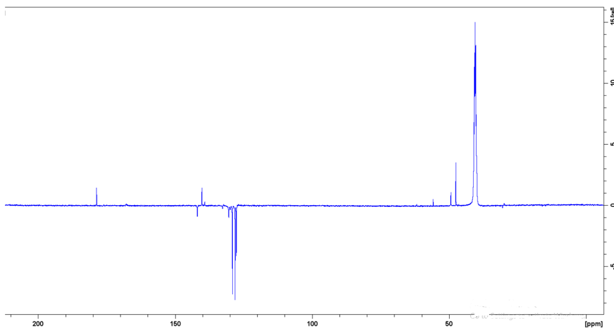
Slika 10. Spektar DEPT-Q NMR tiosemikarbazona P6 snimljen u \text{DMSO-d}_6 pri 298K.
