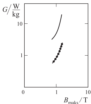
Slika 4. Usporedba gubitaka u jezgri ( G ) za konvencionalnu Fe3\%Si slitinu (puna linija), amorfnu slitinu Fe_{82}B_{10}Si_8 (kružići) iste debljine pri sinusnoj indukciji magnetskog polja B frekvencije 60 Hz.
