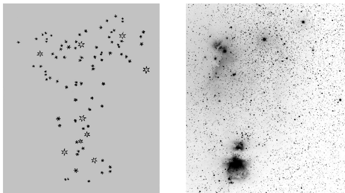
Slika 3. Gdje je god Galileo uperio svoj teleskop u vidnom polju su izranjale zvijezde, nevidljive golim okom. Galilejev crtež pojasa i mača u zvjezdu Orionu (lijevo) i suvremena digitalna slika istog područja (desno).
