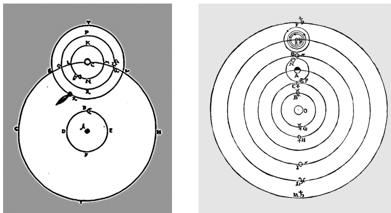
Slika 5. Tychov model svijeta kao svojevrsni kompromis između geocentričnog i heliocentričnog sustava. Zemlja je nepomična, Mjesec i Sunce gibaju se oko Zemlje, dok se planete gibaju oko Sunca. Znameniti komet iz 1577. godine također je naznačen u Tychovom modelu (lijevo). Galilejev model isključivo je heliocentrični, poput Copernicusovog. Novi planeti koji se gibaju oko planeta Jupitera također su naznačeni. Otkrićem Urana i Neptuna, u 18., odnosno 19. stoljeću, Sunčev planetarni sustav je upotpunjen, barem što se tiče planeta (desno).
