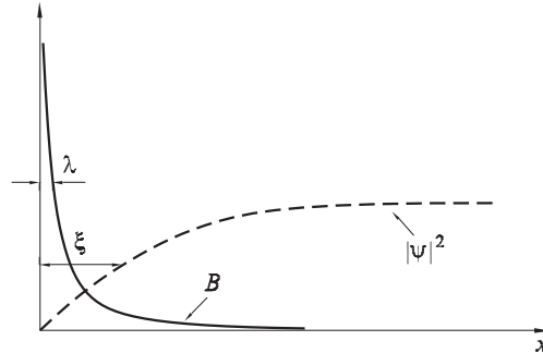
Slika 6. Raspodjela gustoće elektrona |\psi(x)|^2 i magnetskog polja B(x) pri površini supravodiča I. vrste u funkciji udaljenosti x od površine.
