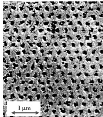
Slika 9. Abrikosovljeva rešetka virova u Nb.
