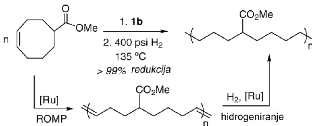
Slika 8. Sinteza polietilena potpomognutom tandemskom katalizom ROMP-hidrogeniranja cikloooktenskih monomera 4
