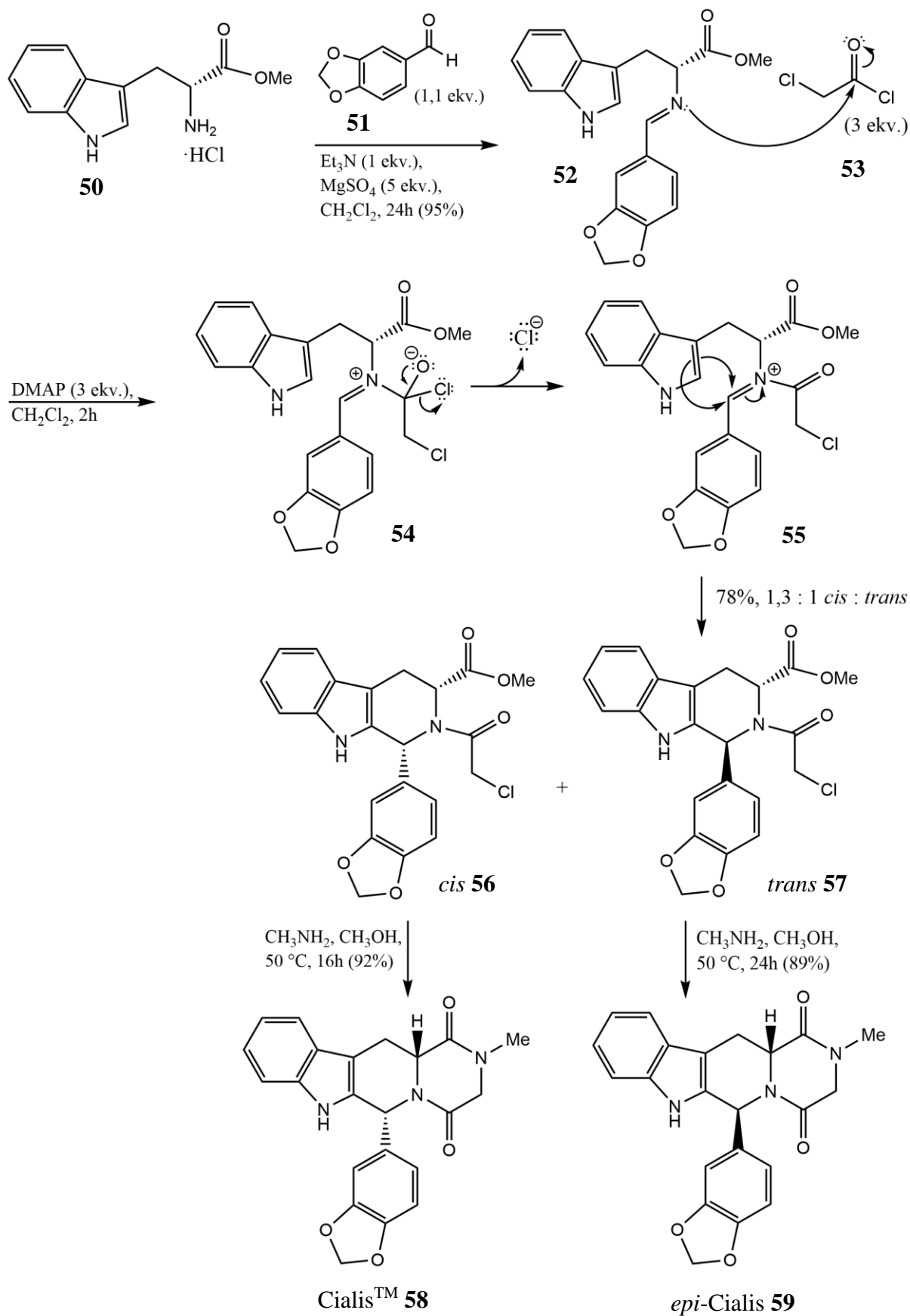
Shema 12. Prikaz reakcije nastajanja Cialisa 58 i epi-Cialisa 59
