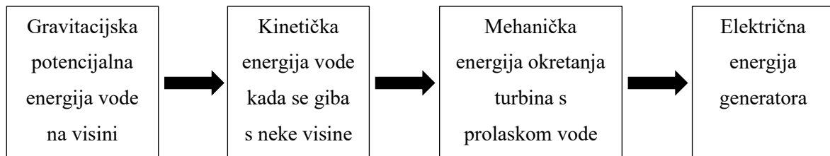
Shema 1: Pretvorbe energije u hidroelektrani.
