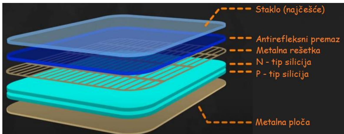
Slika 5: Struktura Si solarne ćelije [21].
