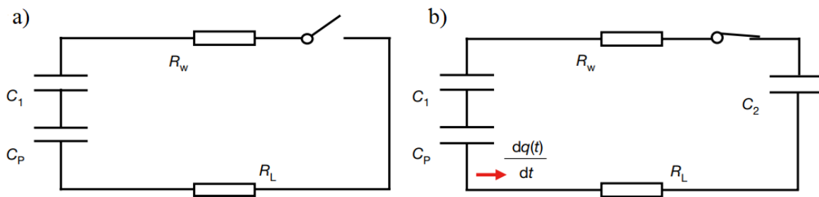
Slika 12: a) Otvoreni strujni krug u kojem se nije formirao kondenzator na granici kapljice vode i aluminijske elektrode ( C_2 ). b) Zatvoreni strujni krug nakon pada kapljice i stvaranja kondenzatora na granici kapljice vode i aluminijske elektrode ( C_2 ). C_p je PTFE kondenzator, C_1 je kondenzator koji nastaje na granici PTFE-a i kapljice vode, R_w i R_L su impedancije kapljice vode i vanjskog strujnog kruga dok razlomak na slici b) označava struju koja poteče krugom (derivacija prenesenog naboja u ovisnosti o vremenu) [24].
