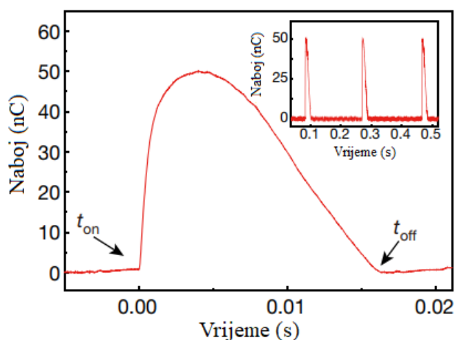
Slika 13: Grafički prikaz ovisnosti naboja o vremenu. Jasno uočavamo da se po gašenju uređaja, naboje vraća na početnu vrijednost. Smanjeni grafički prikaz u gornjem desnom kutu pokazuje istu stvar s povećanjem vremenske skale gdje je vidljivo ponašanje naboja prilikom paljenja i gašenja uređaja [24].
