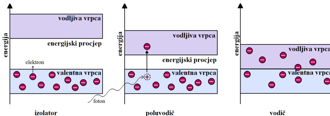
Slika 3: Razlika između energetske procjepa izolatora, poluvodiča i vodiča. [18]
