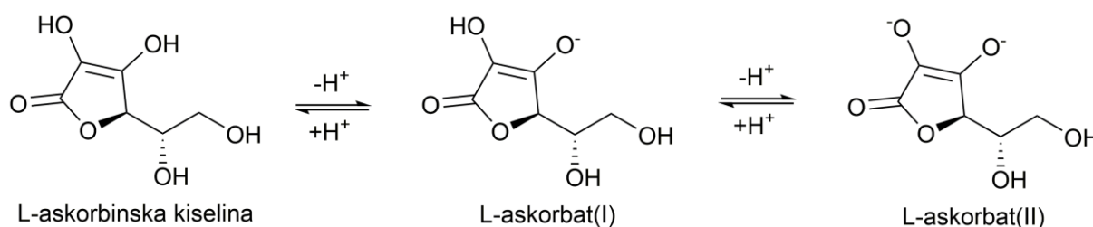
Slika 5. Disocijacija L-askorbinske kiseline u vodi izrađeno u programu ChemDraw
