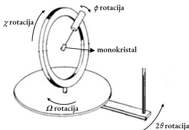
Slika 10. Shema goniometra i goniometarske glave s držačem, slika preuzeta i prilagođena prema izvoru 20
