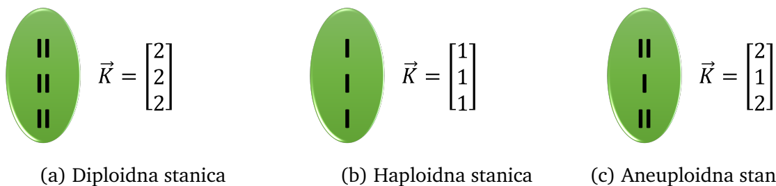
Slika 2.3: Primjeri stanica i njihovih kariotipa. Stanice su prikazane u obliku zelenih ovala dok su kromosomi označeni crnim štapićima. Radi jednostavnosti sheme stanice imaju samo 3 kromosoma, a razlikuju se po broju kopija. (a) Diploidna stanica. Sva tri kromosoma imaju dvije kopije ( c_1 = c_2 = c_3 = 2 ). (b) Haploidna stanica. Sva tri kromosoma imaju jednu kopiju ( c_1 = c_2 = c_3 = 1 ). (c) Aneuploidna stanica. Prvi i treći kromosom imaju dvije kopije ( c_1 = c_3 = 2 ), dok drugi kromosom ima jednu kopiju ( c_2 = 1 ).
