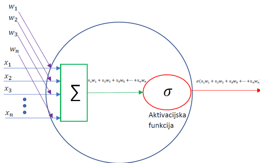
Slika 4.11: Model neurona.
