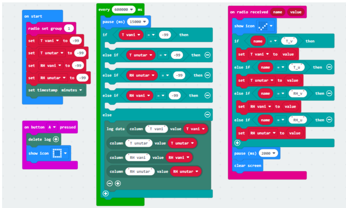
Slika 4.2.11 Kompletan kod prijemnika.
