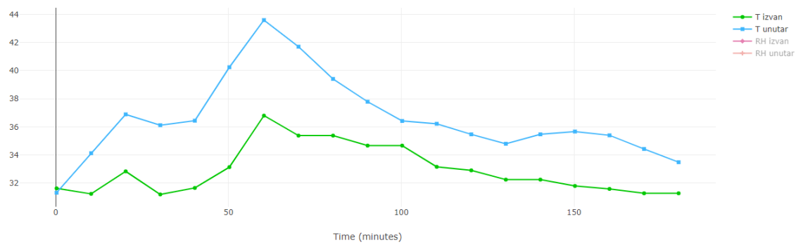
Slika 5.1.11 Grafički prikaz temperatura unutar i izvan platenika u vremenu.
