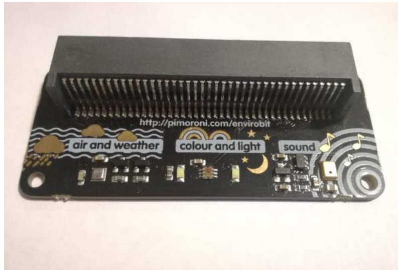
Slika 4.2 Enviro:bit pločica. Pozicije pojedinih senzora naznačene su na pločici.
