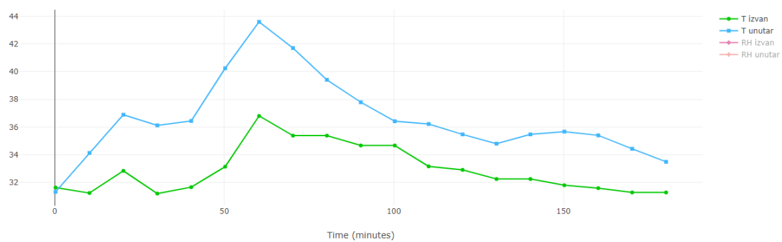
Slika 5.1.11 Grafički prikaz temperatura unutar i izvan plastenika u vremenu.
