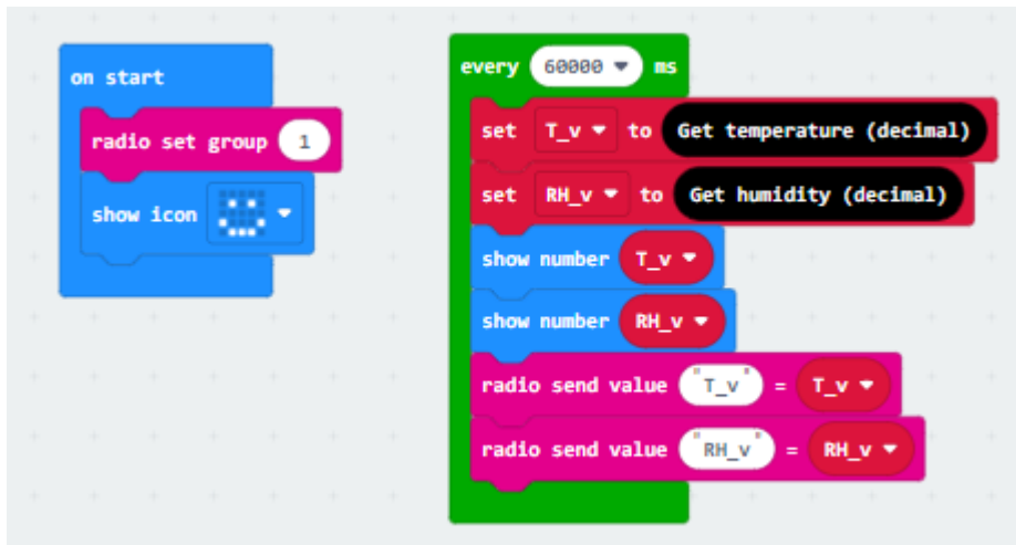
Slika 4.2.4 Kod za odašiljač (vanjski uvjeti) .
