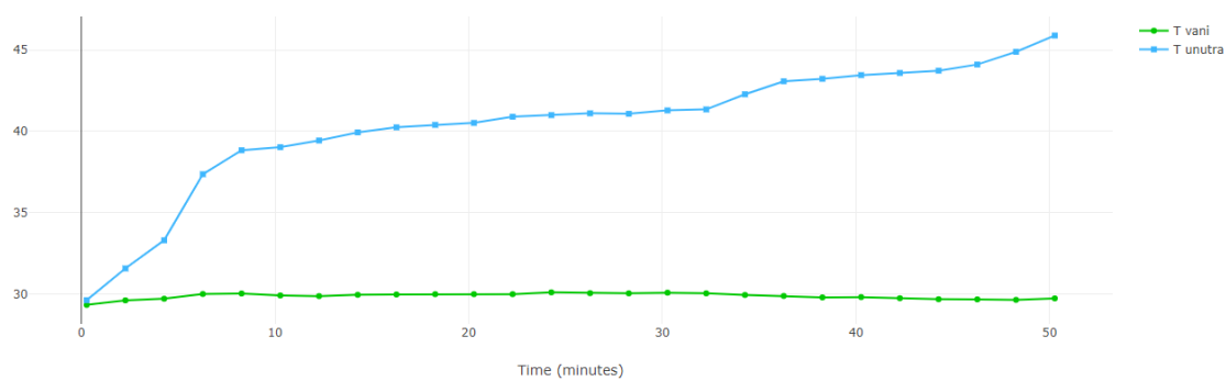
Slika 5.3.3 Odnos temperatura unutar i izvan plastenika za vrijeme mjerenja.
