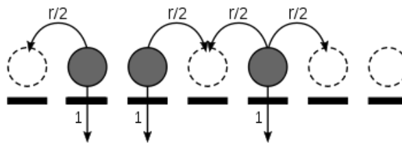
Slika 4.1: Kontaktni proces na 1D rešetci. Popunjene pozicije (zaraženi pojedinci) su označene sivim krugovima, dok su prazne pozicije (zdravi pojedinci) označene isrtanim krugovima. Popunjene pozicije mogu aktivirati prazne susjedne pozicije vjerojatnošću r/2 ili postati neaktivne vjerojatnošću 1. Preuzeto iz [12].
