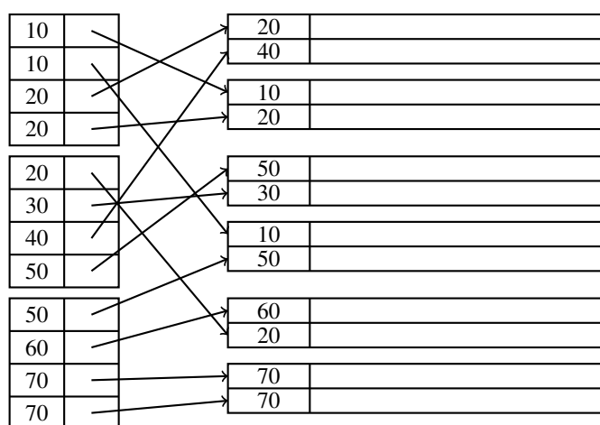
Slika 4.4: Sekundarni indeks
