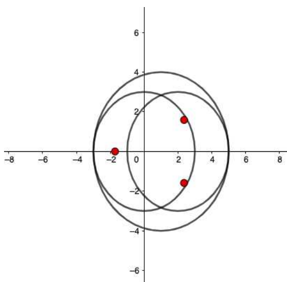
Slika 3.1: Svojtvene vrijednosti matrice X
