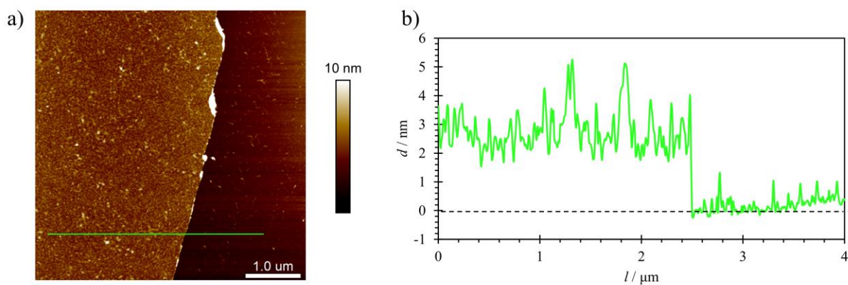
Slika 32. a) AFM snimka poroznog (\text{PAH}_1/\text{PAA}_h)_5 višesloja pripravljenog pri \text{pH} = 5 i b) visinski profil područja označenog zelenom linijom na slici pod a)
