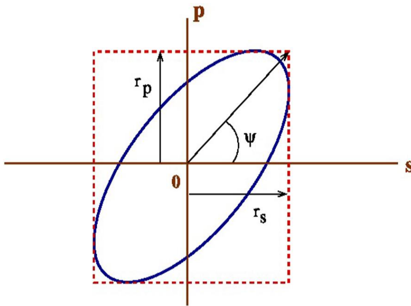
Slika 10. Eliptično polarizirano zračenje 28
