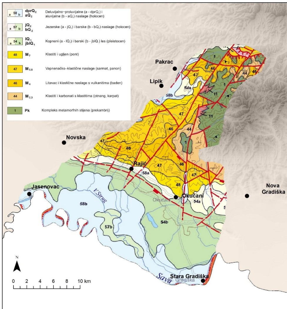
Slika 2. Geološka karta
