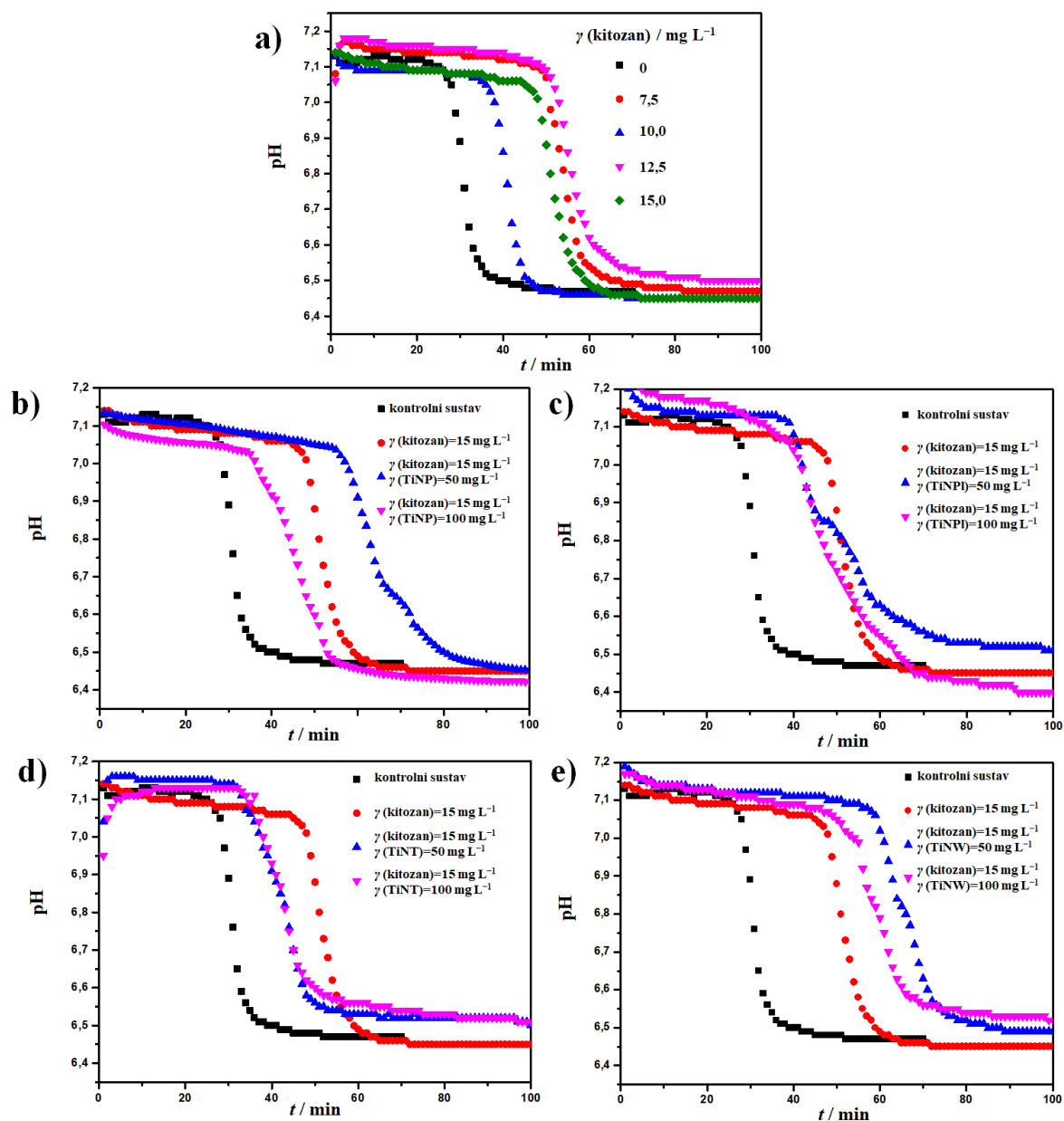
Slika 72. Reprezentativne pH krivulje a) sustava koji sadrži samo kitozan i sustava u kojima su, uz 15 mg mL -1 kitozana, dodane b) TiO 2 nanočestice (TiNP), c) TiO 2 nanopločice (TiNPI), d) titanatne nanocjevčice (TiNT) i e) titanatne nanožice (TiNW) koncentracije 50 i 100 mg mL -1 . c_{\text{poč}}(\text{CaCl}_2) = c_{\text{poč}}(\text{Na}_2\text{HPO}_4) = 4 \cdot 10^{-3} \text{ mol dm}^{-3} pri 25 °C i \text{pH}_{\text{poč}} = 7,4 .
