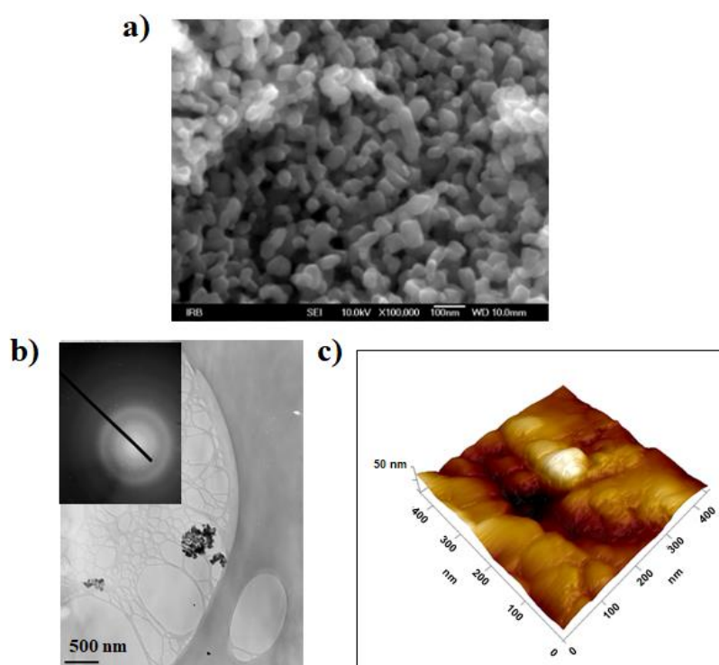
Slika 25. a) SEM, b) TEM i c) AFM mikrografije \text{TiO}_2 nanopločica.
