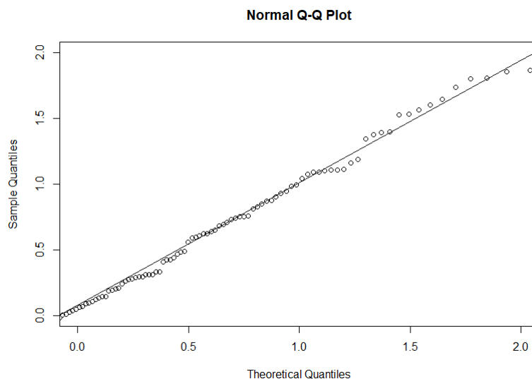
Slika 3.2: Normalni vjerojatnosni graf
