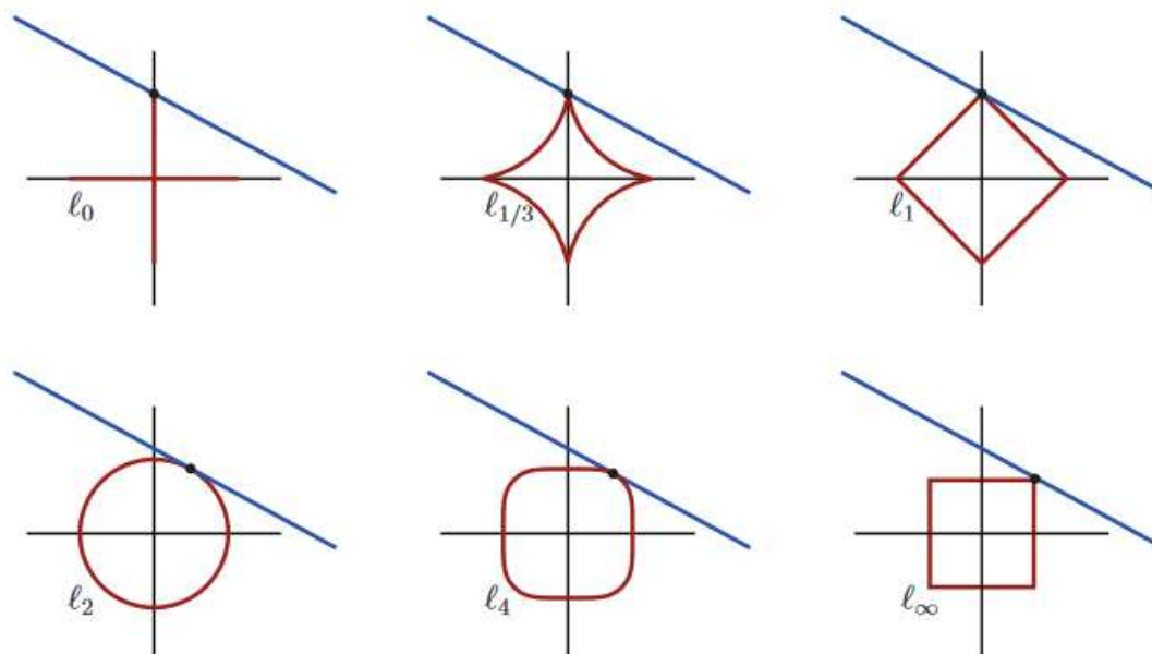
Slika 2.1: Prikazane su točke s najmanjom normom koje pripadaju nekom skupu za različite l_p norme. Plava linija prikazuje rješenja nekog neodređenog sustava jednačbi, a crvene krivulje najmanje kugle p norme koji dodiruje skup rješenja
