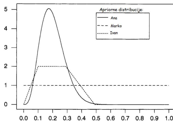
Slika 3.1: Apriorne distribucije
