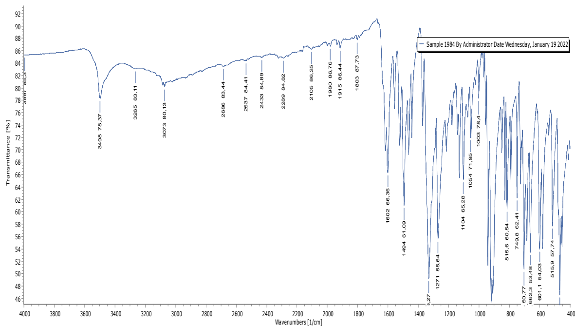
Slika D15. IR spektr smjese kompleksa [\text{MoO}_2(\text{L})(\text{MeOH})] i [\text{MoO}_2(\text{L})(\text{H}_2\text{O})] .
