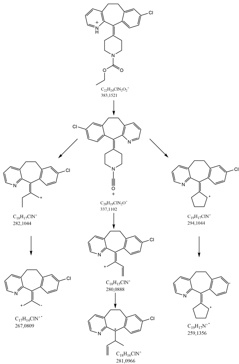
Slika 26. Fragmentacijska shema loratadina
