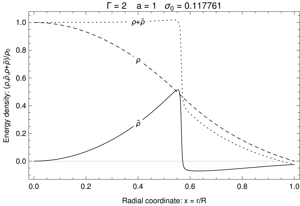
Slika 6.3: Prikazano je ponašanje gustoće energije za konkretnu zvijezdu sa središnjom gustoćom \sigma_0 = 0.117761 u slučaju f(T) = T + \alpha T^2/2 gdje je a = \alpha \lambda^{-2} = 1 . Vidljiv je strmi pad \mathring{G}^{tt} komponente Einsteinovog tenzora blizu polovice polumjera zvijezde, te spajanje na vakuum. Gustoća energije politropskog fluida se neznatno razlikuje od onoga u općoj teoriji relativnosti za \Gamma = 2 .
