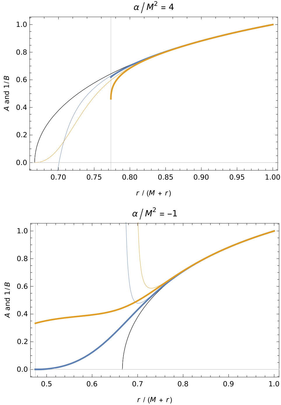
Slika 5.3: Numeričko vakuumsko rješenje u f(T) = T + \frac{\alpha}{2}T^2 za \alpha/M^2 = 4 (gornji graf) i za \alpha/M^2 = -1 (donji graf): Funkcije numeričkog rješenja A (debela plava linija) i 1/B (debela narančasta linija), funkcije perturbativnog rješenja A (tanka plava linija) i 1/B (tanka narančasta linija), funkcije A = 1/B Schwarzschildovog rješenja (tanka crna linija). Crne uspravne linije označavaju položaj singularne sferne plohe.
