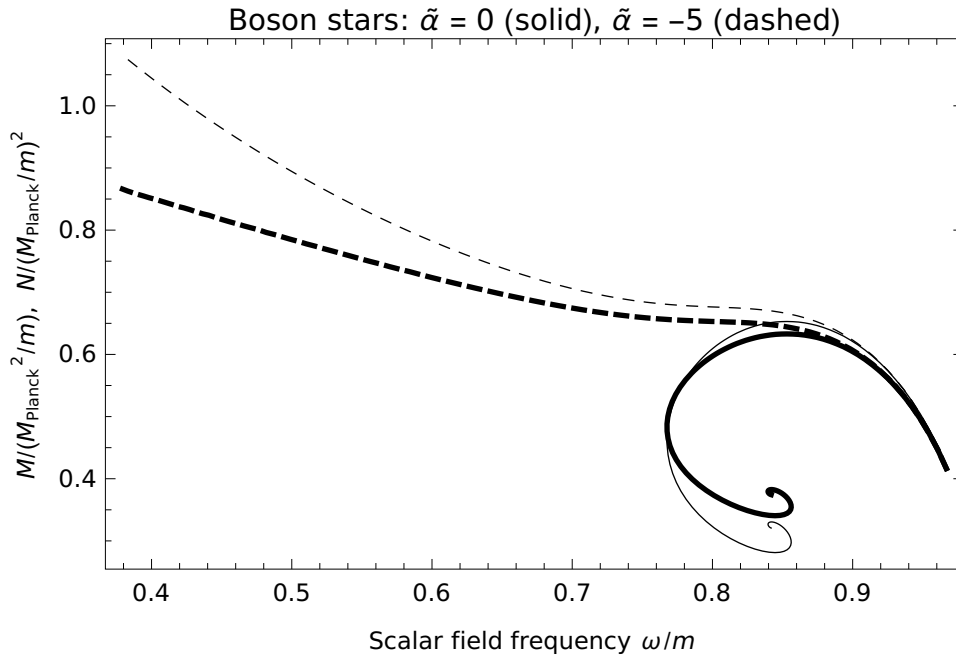
Slika 6.8: Predstavljene su vrijednosti mase i broja čestica u ovisnosti o frekvencijama \omega/m za \tilde{\alpha} = 0 i \tilde{\alpha} = -5 . Isprekidane linije predstavljaju masu i broj čestica u f(T) gravitaciji, te analogno tome pune linije predstavljaju masu i broj čestica u općoj teoriji relativnosti. Deblje linije su mase u jedinicama M_{Plank}^2/m , a tanje linije su broj čestica u M_{Plank}^2/m^2 .
