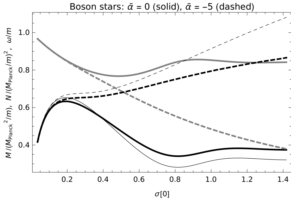
Slika 6.7: Predstavljene su vrijednosti mase, broja čestica i frekvencije skalarnog polja u ovisnosti o središnjoj gustoći skalarnog polja \sigma_0 za \tilde{\alpha} = 0 i \tilde{\alpha} = -5 . Isprekidane linije predstavljaju masu, broj čestica i frekvenciju u f(T) gravitaciji, te analogno tome pune linije predstavljaju masu, broj čestica i frekvenciju u općoj teoriji relativnosti. Deblje linije su mase u jedinicama M_{\text{Planck}}^2/m , tanje linije su broj čestica u M_{\text{Planck}}^2/m^2 , a sive linije su frekvencije \omega/m .
