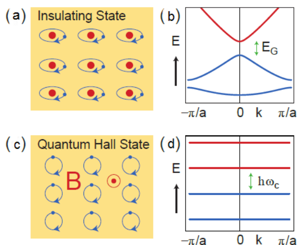
Slika 3.2: a), b) Prikaz standardnog izolatora i pripadnog energetskog spektra s disperzijom. c), d) Stanje kvantnog Hallovog efekta u jakom magnetskom polju i prikaz degeneriranih Landau razina u spektru - preuzeto iz [10].
