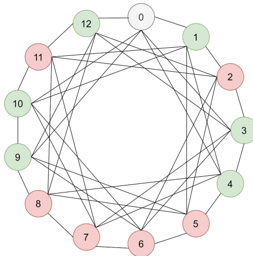
Slika 12: Graf QR(13) s označenim susjednim (zeleno) i nesusednim (crveno) vrhovima od vrha 0.
