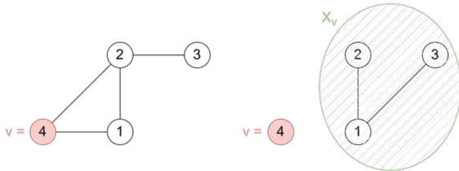
Slika 4: Graf X i X_v , za v = 4 .
