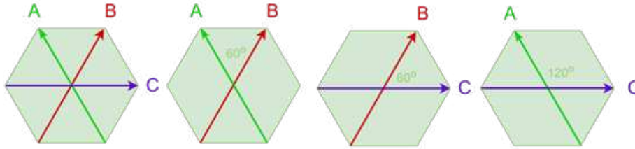
Slika 2: Primjer triju ekvianularnih pravaca u \mathbb{R}^2 reprezentiranih jediničnim vektorima (O, A) , (O, B) i (O, C) .
