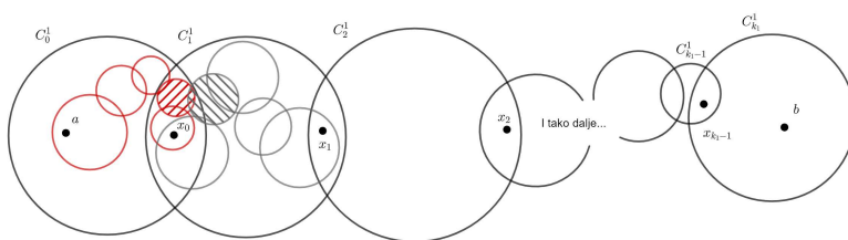
Slika 4.3: U ovoj ilustraciji istaknuti su lanac \mathcal{D}^0 i \mathcal{D}^1 , a karike D_{n_0}^0 i D_{p_1}^1 su išarane.
