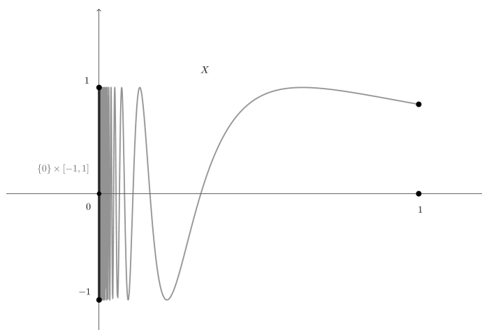
Slika 2.1: Topološka sinusoida, s podskupom \{0\} \times [-1, 1] označenim crnom bojom i podskupom \{(x, \sin \frac{1}{x}) \mid x \in \langle 0, 1] \} označenim sivom bojom.
