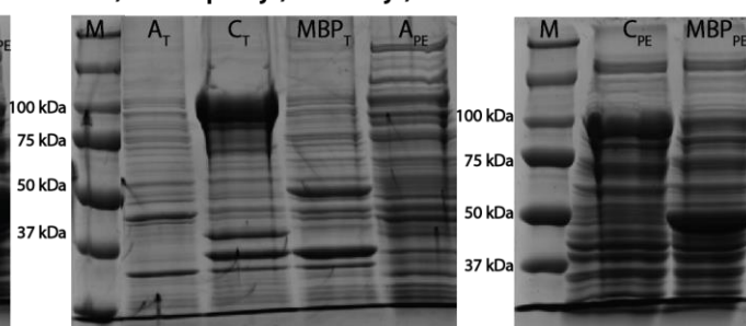
Slika D10. SDS-PAGE analiza ekspresije krnjih oblika BmIleRS2 fuzioniranih s GST-privjeskom na 16 °C i 37 °C uz 0,25 mmol dm -3 IPTG, razbijanje stanica uz BugBuster . ON označava ekspresiju preko noći, A, B, C krnje IleRS2 fuzionirane s GST, M marker, T u indeksu talog, a PE proteinski ekstrakt. Korišten je marker Precision Plus Protein Standards Unstained ( Bio-Rad ).
