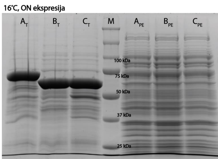
Slika 4.8. SDS-PAGE analiza ekspresije krnjih oblika BmIleRS2 na 16 \text{ }^{\circ}\text{C} uz 0,1 \text{ mmol dm}^{-3} IPTG i razbijanje stanica uz BugBuster . ON označava ekspresiju preko noći, A, B, C krnje IleRS2, M marker, T u indeksu talog, a PE proteinski ekstrakt. Korišten je marker Precision Plus Protein Standards Unstained ( Bio-Rad ).
