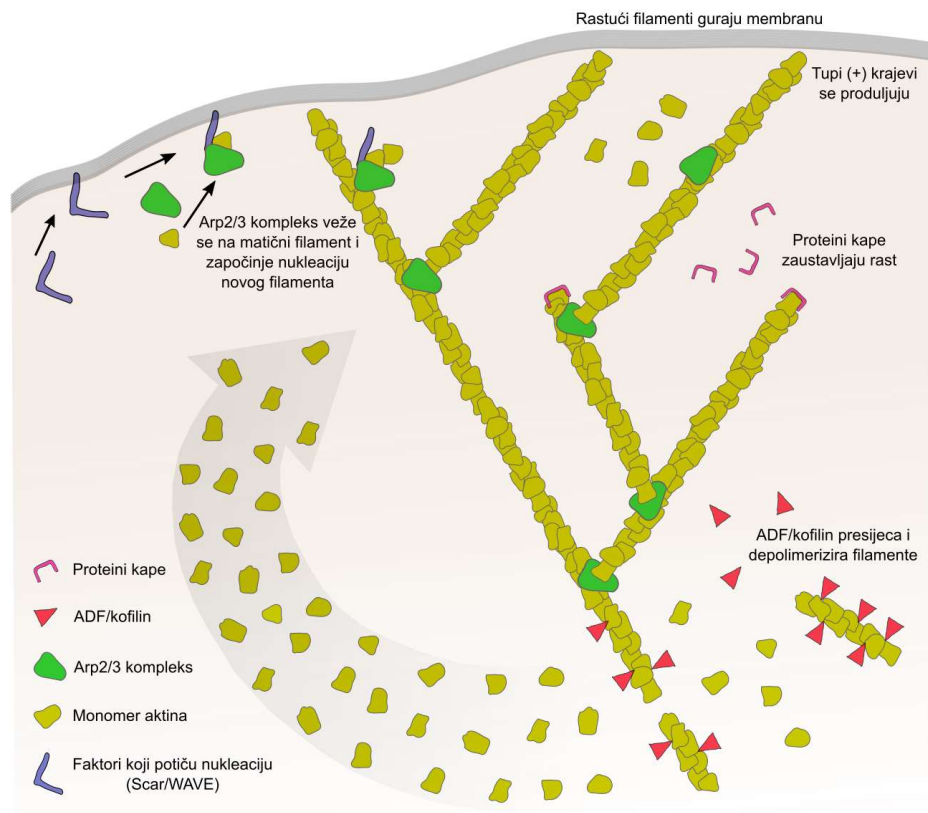
Slika 1-2. Stvaranje razgranate mreže aktina. Aktivacijom kompleksa Arp2/3 i vezanjem za matični filament započinje nukleacija novog filamenta, koji gura membranu prema naprijed. Neograničeni rast filamenata sprječavaju proteini kape, a cijepanje i depolimerizaciju filamenata obavlja ADF/kofilin, te tako oslobađa monomere za recikliranje. Prilagođeno prema (Pollard and Cooper, 2009).
