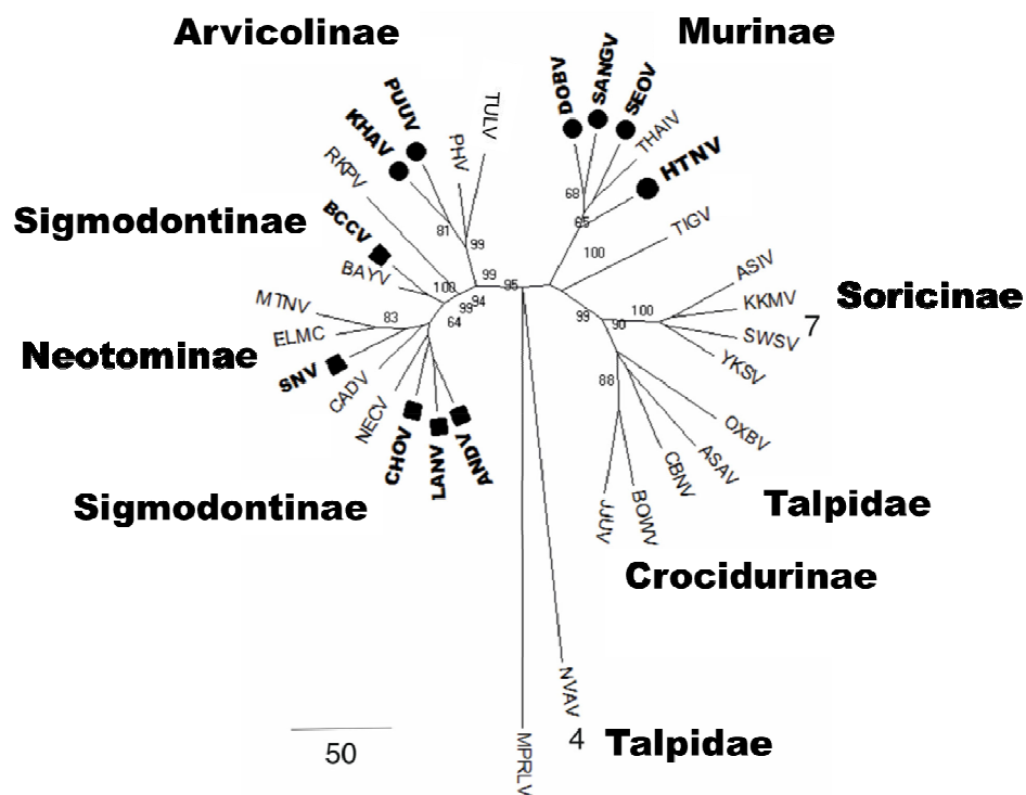
Slika 4. Filogenetsko stablo ortohantavirusa, na bazi potpunog S segmenta. Ljudski patogeni su označeni podebljanim slovima (● – HVBS, ■ – HCPS). Modificirano prema Kabwe et al. 2020.
