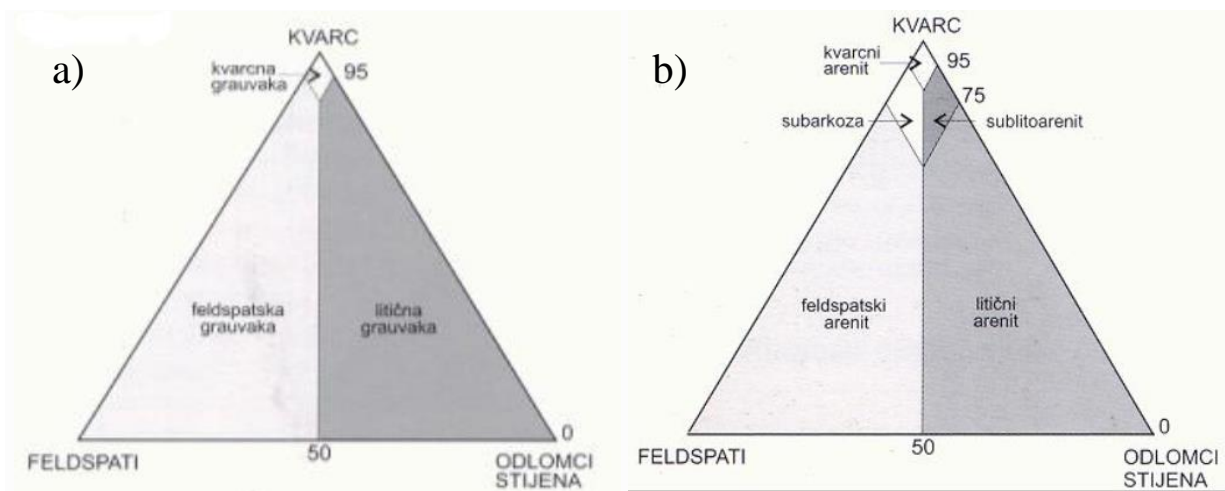
Slika 8. Q-F-LF trokomponentni dijagrami klasifikacije pješčenjaka na a) grauivake i b) arenite ovisno o udjelu matriksa u stijeni te podjela istih unutar pojedinog dijagrama prema postotku detektiranog detritičnog sadržaja izvedeno prema PETTIJOHNU et al. (1987)
