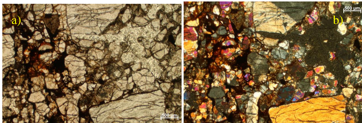
Slika 34. a) Fotomikrografija uzorka s točke T5 s povećanjem 2,5 puta bez analizatora i b) s analizatorom. Vidljive različite veličine zrna, kao i mnoštvo zrna olivina.
