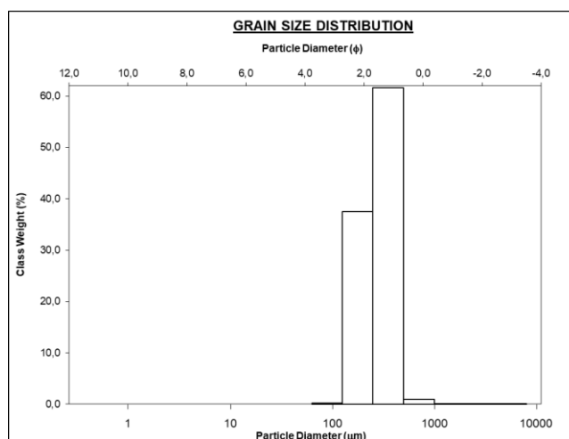
Slika 15: Histogram uzorka SAH 7.
