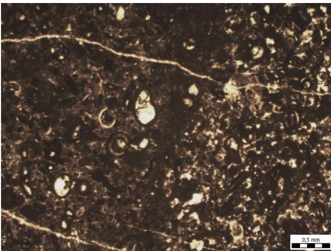
Slika 14. Foraminifersko-peloidni vekston do pekston s cijanobakterijama Decastronema kotori (RADOČIĆ) te Thaumatoporella parvovesiculifera (RAINERI), SAV-11.
