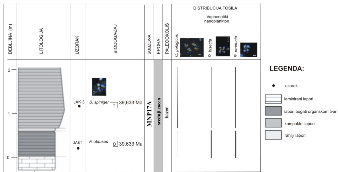
Slika 19. Prikaz biodogađaja u stupu Jakomići II na temelju kojih je određena baza podzone MNP17A
