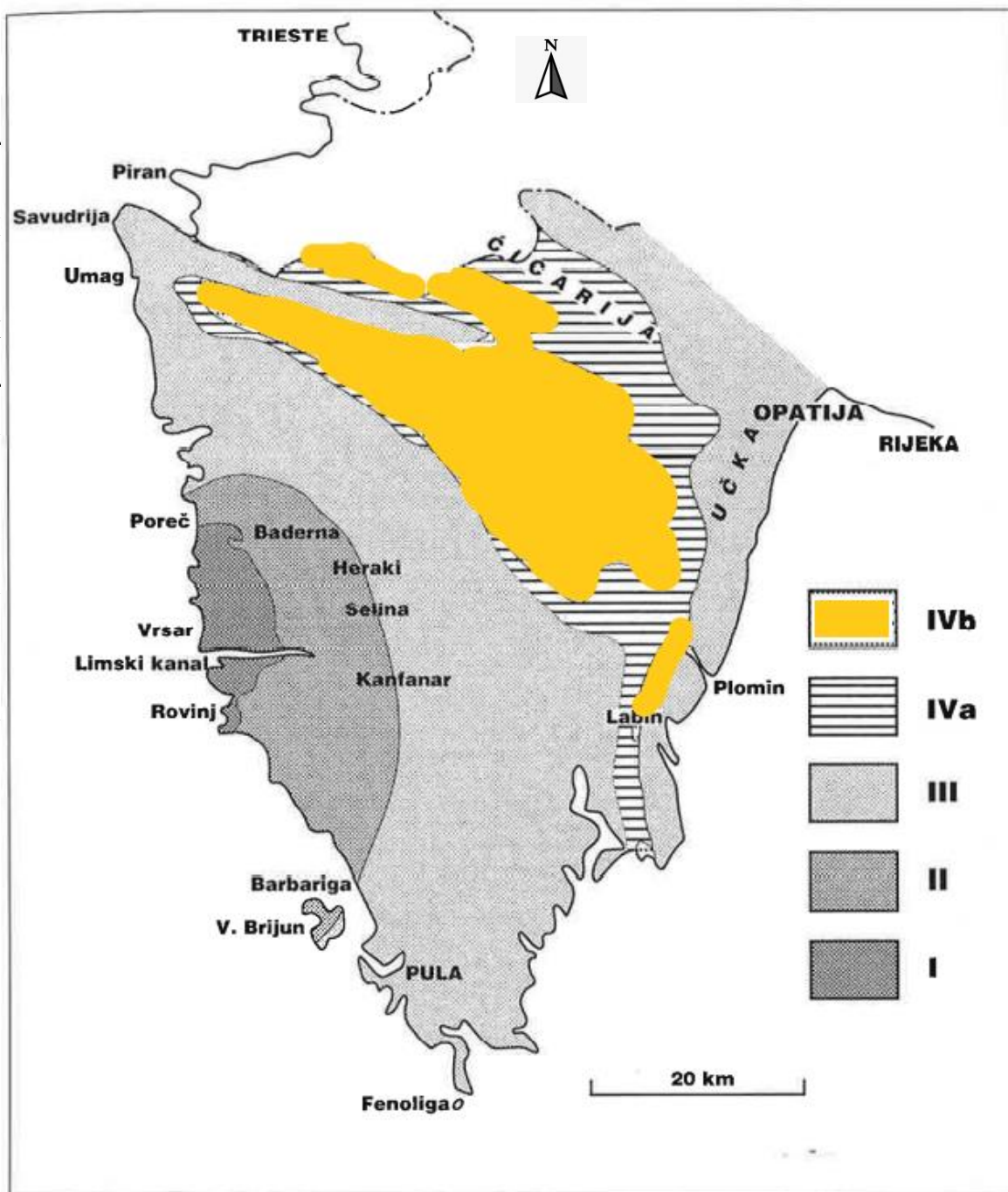
Slika 1. Pojednostavljena litosekvencijska karta Istre s prikazanim prostiranjem naslaga prepoznatih megasekvencama i žutom bojom istaknum prijelaznim naslagama i flišem. Legenda: I) bat-donji kimeridž; II) gornji titon-gornji apt; III) gornji alb-donji kampan; IV) paleocen-eocen: a) foraminiferski vapnenci i b) prijelazne naslage i fliš (žuta boja) (preuzeto i modificirano prema VELIĆ i sur., 1995)
