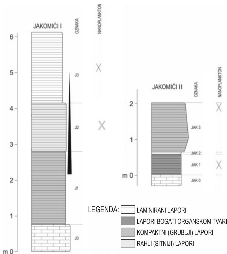
Slika 4. Shematski prikaz geoloških stupova Jakomići I i Jakomići II
