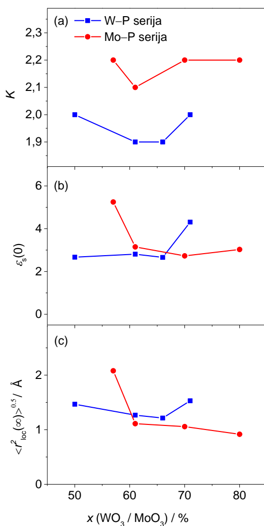
Slika 43. Trendovi ovisnosti (a) parametra K , (b) plateau-a skalirane permitivnosti, \varepsilon_s(0) , i (c) prostornog doseg lokaliziranih skokova polarona, \langle r_{loc}^2(\infty) \rangle^{0.5} , o udjelu \text{WO}_3 i \text{MoO}_3 u serijama stakala x\text{WO}_3-(100-x)\text{P}_2\text{O}_5 i x\text{MoO}_3-(100-x)\text{P}_2\text{O}_5 , x = 50-80 %.
