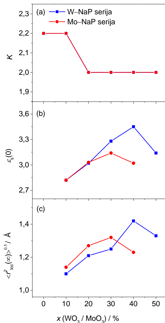
Slika 75. Trendovi ovisnosti (a) parametra K , (b) plateau-a skalirane permitivnosti, \varepsilon_s(0) , i (c) prostornog dosega lokaliziranih skokova iona natrija, \langle r_{loc}^2(\infty) \rangle^{0.5} , o udjelu WO_3 i MoO_3 u serijama stakala xWO_3-40Na_2O-(60-x)P_2O_5 i xMoO_3-40Na_2O-(60-x)P_2O_5 , x = 0-50 %.
