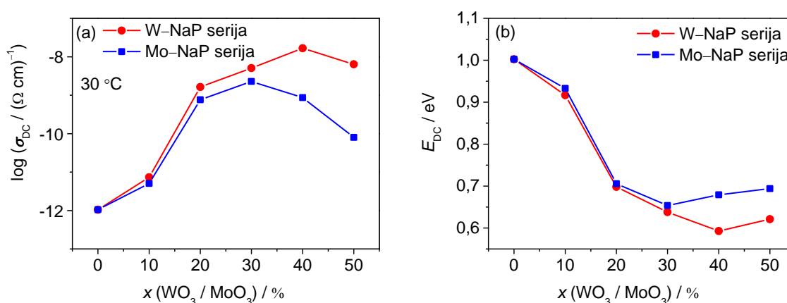
Slika 67. Ovisnost (a) DC provodnosti na 30^\circ \text{C} i (b) energije aktivacije za DC provodnost o množinskom udjelu \text{WO}_3 i \text{MoO}_3 u serijama stakala x\text{WO}_3-40\text{Na}_2\text{O}-(60-x)\text{P}_2\text{O}_5 i x\text{MoO}_3-40\text{Na}_2\text{O}-(60-x)\text{P}_2\text{O}_5 , x = 0-50 %.
