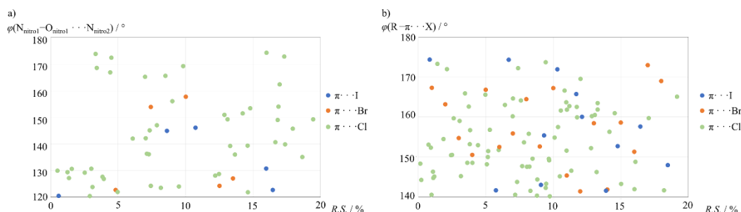
Slika 14. Dijagrami raspršenja ovisnosti kuta i relativnog skraćenja pnikogenske i halogenske veze u višekomponentnim kristalima koji sadrže molekule s halogenim atomima i nitro skupinom, s \pi -sustavom kao akceptorom halogenske veze.
