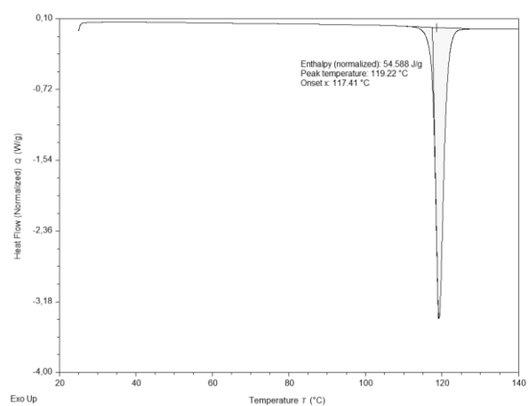
Slika D75. DSC krivulja (nba4Ian)(135tfib).
