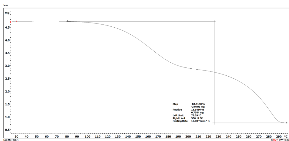
Slika D54. Termogram (nba4Ian)(13t).
