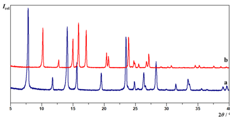
Slika D8. Usporedba difraktograma: a) nba , b) produkt dobiven iz otopine nba i 3Clan u MeOH.
