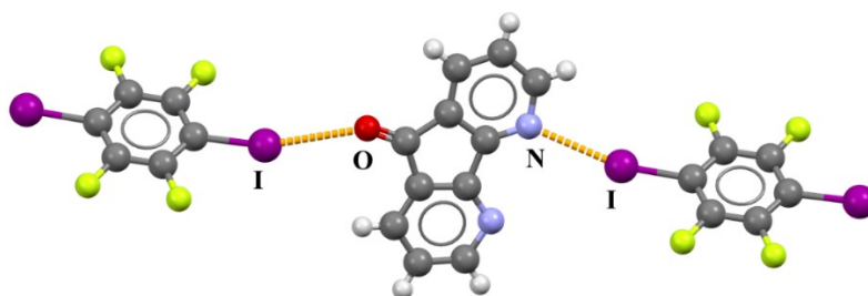
Slika 5. Primjer ditopične akceptorske molekule 1,10-fenantrolin-5-diona povezane halogenkim vezama N...I i O...I u strukturi EXIFAT. 40
