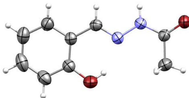
Slika 9. Molekulska struktura hidrazonskog liganda pripravljenog iz acetohidrazida 37 ;
