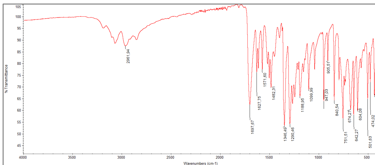
Slika D4. IR spektar liganda H_2L^2
