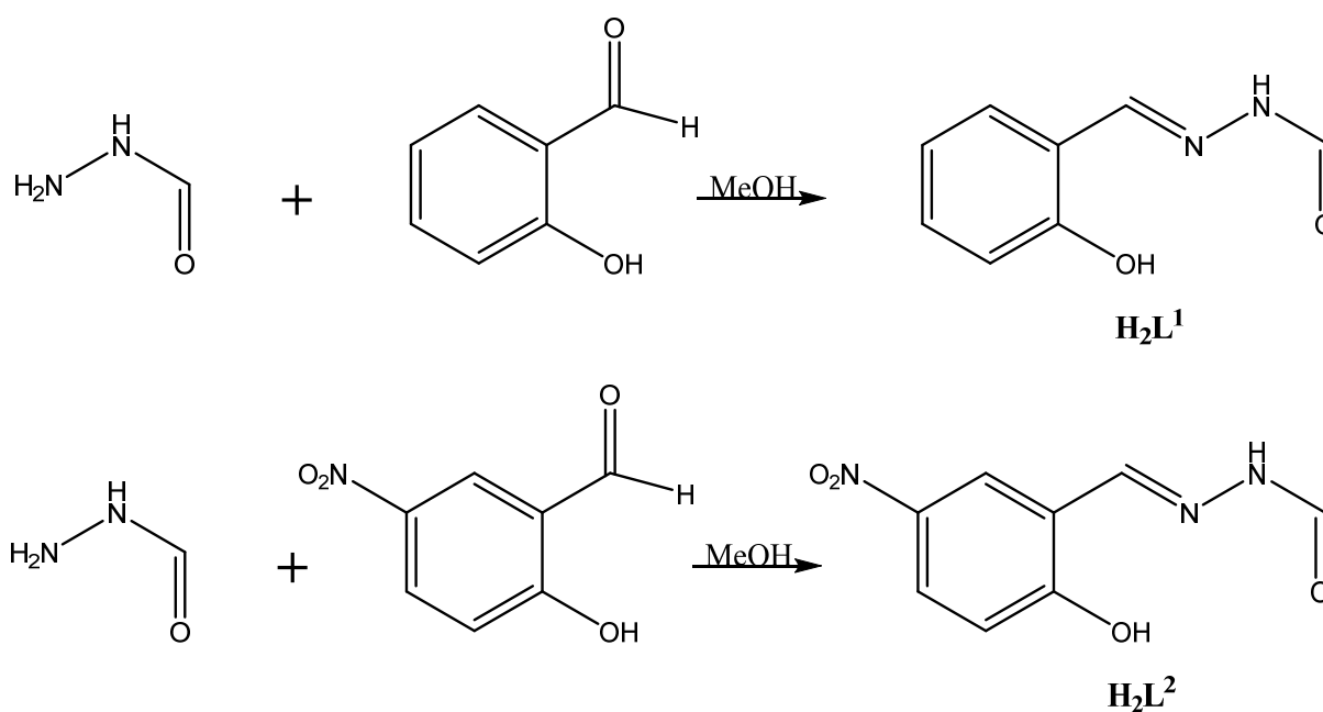
Shema 7. Sinteza hidrazonskih liganada ( \text{H}_2\text{L}^1 ; \text{H}_2\text{L}^2 )
