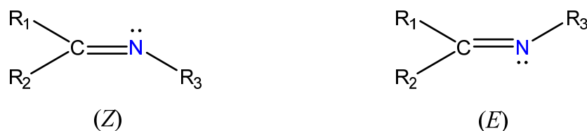
Slika 1. Prikaz općenite strukture Schiffove baze
