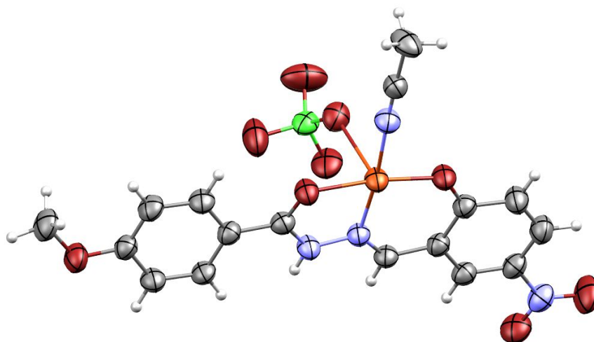
Slika 5. Molekulska struktura mononuklearnog kompleksnog spoja [\text{Cu}(\text{HabsNO}_2)(\text{CH}_3\text{CN})(\text{ClO}_4)]_2^{27} ; Mercury – POV-Ray prikaz
