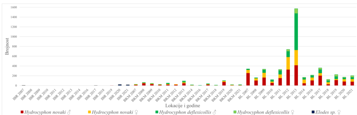
Slika 13 Brojnost porodice Scirtidae na tri lokacije u razdoblju od 2007. do 2021. Skraćenice lokacija: IBR: Izvor Bijele rijeke, BKM: Barijera Kozjak Milanovac, BL: Barijera Labudovac.
