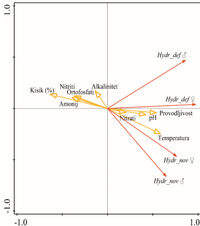
Slika 38 PCA analiza odnosa vodenih kornjaša i fizikalno-kemijskih pokazatelja vode na lokaciji Barijera Labudovac. Skraćenice: Hydr_nov : Hydrocyphon novaki , Hydr_def : Hydrocyphon deflexicollis .
