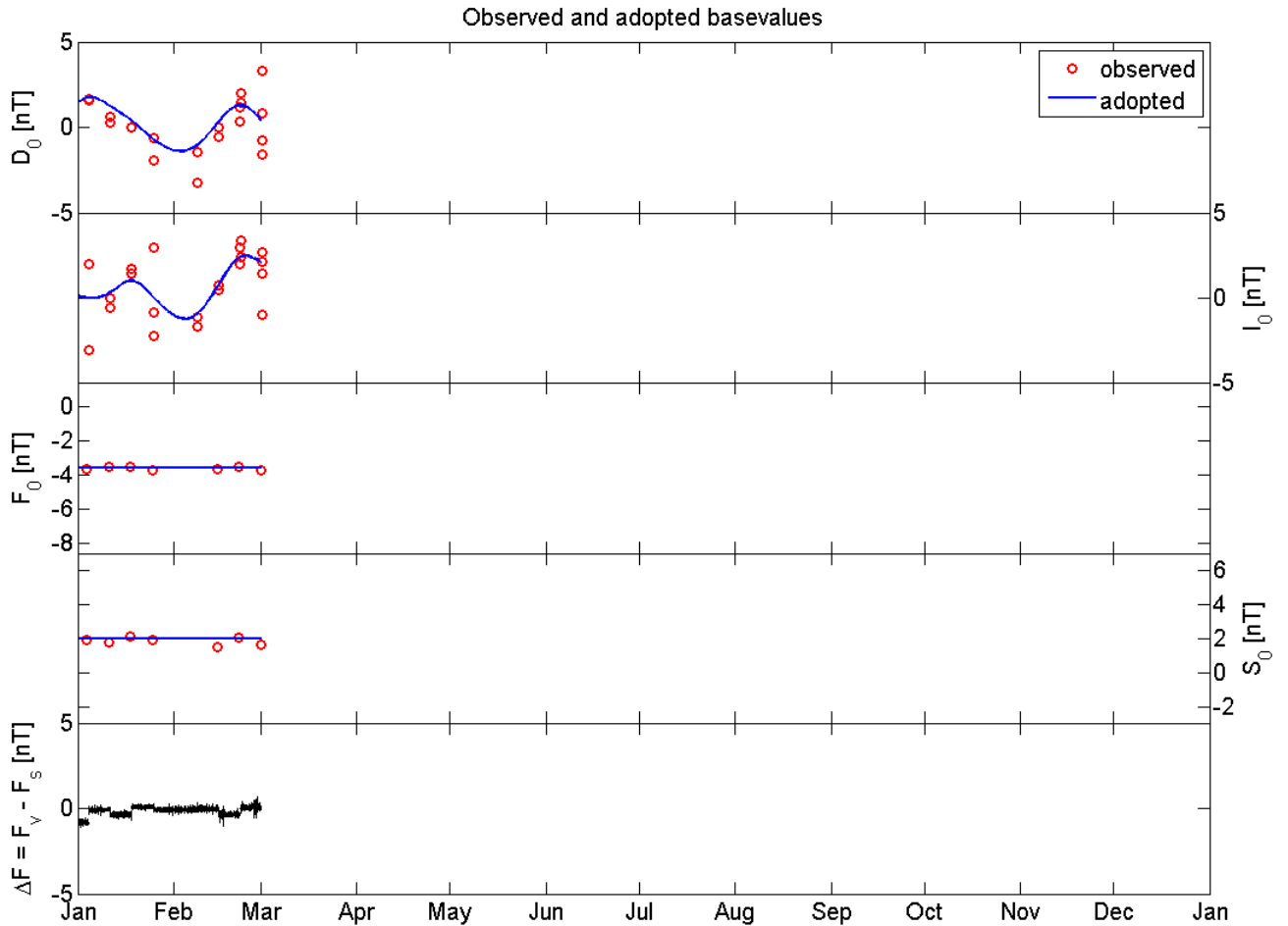
Slika 2.2 – Opažene ( engl. observed ) i prilagođene ( engl. adopted ) kalibracijske vrijednosti za DIDD variometar. Na slici su također prikazani rezultati motrenja s početka ožujka koji su korišteni u izračunu kalibracijskih krivulja za veljaču.
