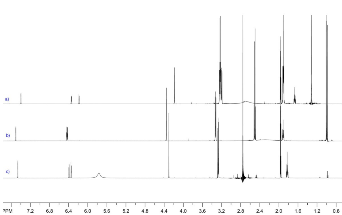
Slika D22. ^1\text{H-NMR} spektar spoja 6 \cdot \text{HI} i a) \text{P}_1\text{pyrr}_3^* \text{t-Bu} , b) \text{Et}_3\text{N} i c) \text{TMG} u ekvimolarnoj količini
